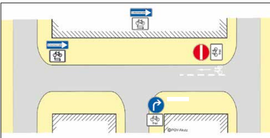
Bild 5b | Weitere Führungsformen des Radverkehrs: für Radverkehr in Gegenrichtung freigegebene Einbahnstraße
